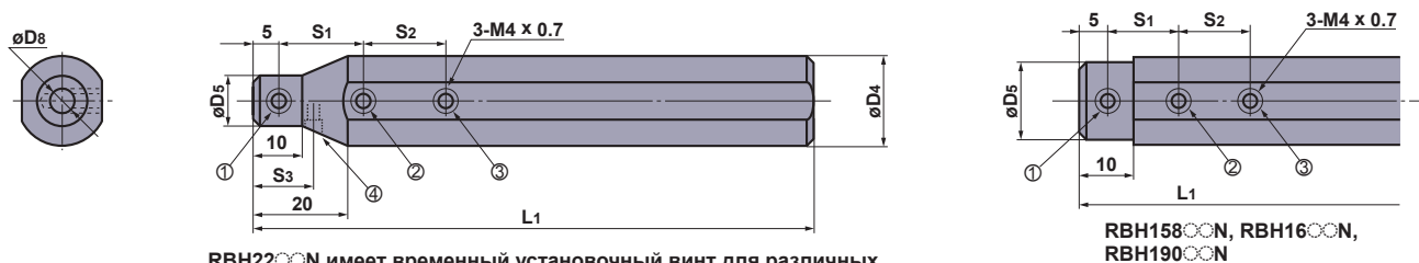
RBH220N имеет временный установочный винт для различных комплектаций станков (изображён под номером 4).
